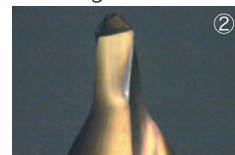
②他社製HSSセンタードリル TiNコーティング
