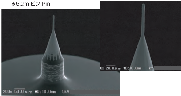
φ5μm ピン Pin
